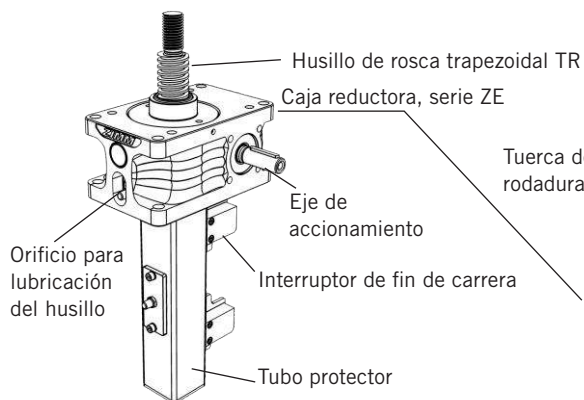
Traslación del husillo (versión S)
