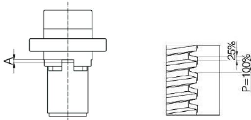
Fig. 20. Tuerca de retención de seguridad SIFA: Dimensión “A” para la comparación en la comprobación del desgaste.
