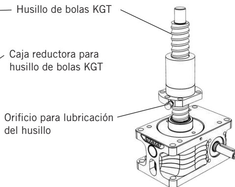
Rotación del husillo (versión R)
