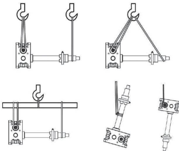
Fig. 5. Ejemplos para el transporte de la versión R
