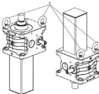
Fig. 6. Tornillos con ojo (1) o tuercas anulares (no incluidos en el volumen de suministro)
