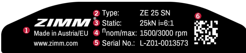
Fig. 3. Ejemplo de una placa de características.
