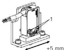
Fig. 17. Ajuste preciso del interruptor de fin de carrera.
