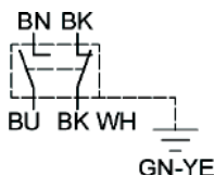
Fig. 15. Esquema de conexiones eléctricas del interruptor de fin de carrera.
