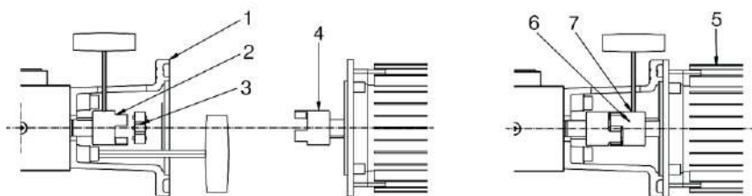
Fig. 13. Montaje del motor
