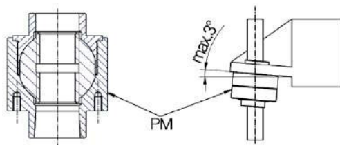
Fig. 10. Excepción: El ángulo de inclinación máximo de la tuerca oscilante (PM) es de 3°; monte todas las demás tuercas sin inclinación.
