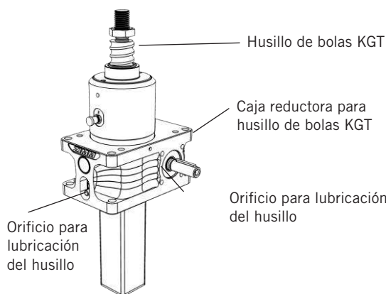
Traslación del husillo (versión S)
