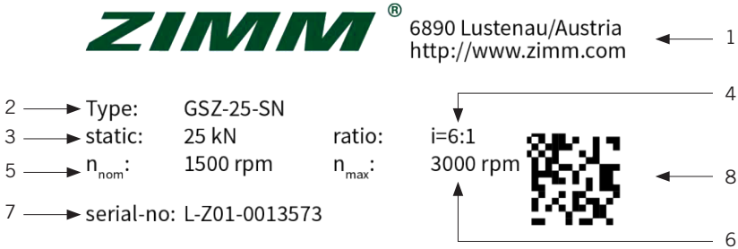
Fig. 2. Ejemplo de una placa de características.
