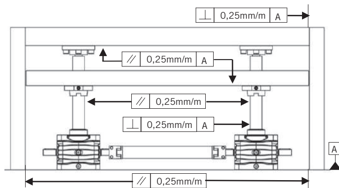
Fig. 8. Planitud, paralelismo y precisión angular.
