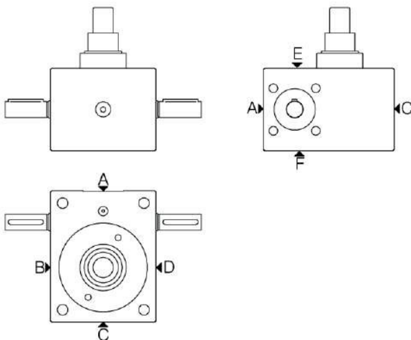
Fig. 1. Visión global del elevador de husillo ZIMM. De A a F: caras laterales del elevador de husillo ZIMM.
