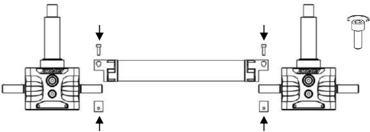
Fig. 12. Montaje de los ejes de transmisión.
