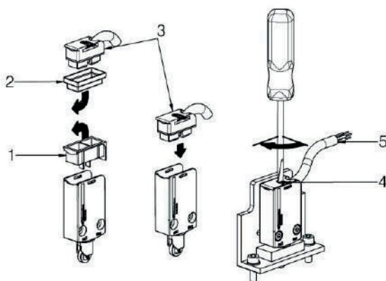
Fig. 14. Montaje de la clavija de conexión en el interruptor de fin de carrera.
