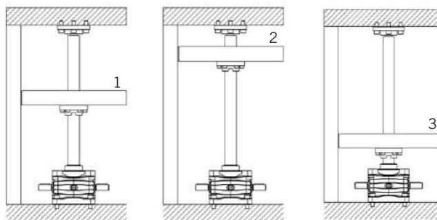
Fig. 19. Elevador de husillo correctamente alineado versión R.
