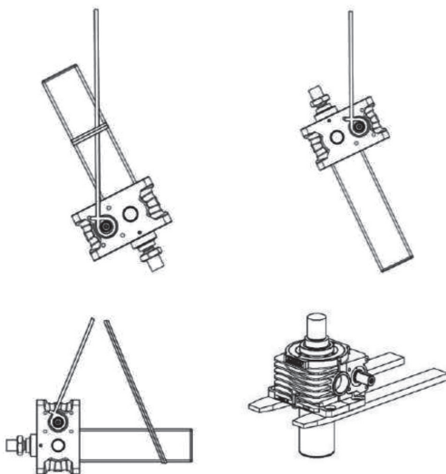
Fig. 4. Ejemplos para el transporte de la versión S
