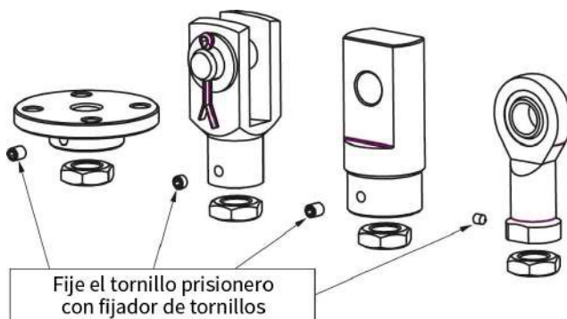
Fig. 9. Fije los accesorios como las bridas de sujección, los cabezales de horquilla, rótula o pivotante después de ajustar la posición.
