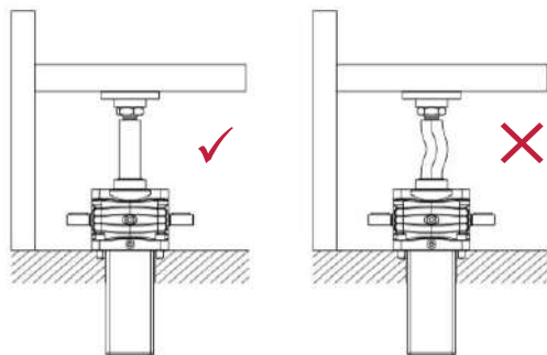
Fig. 7. Esfuerzo lateral en el husillo no permitido.
