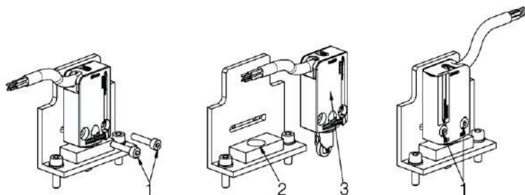
Fig. 16. Giro de la salida del cable del interruptor de fin de carrera.
