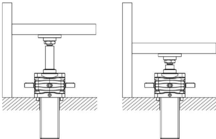
Fig. 18. Elevador de husillo correctamente alineado versión S.
