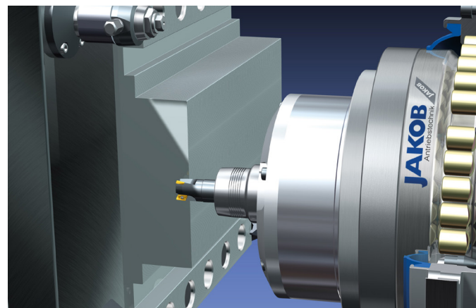
Colisión radial
