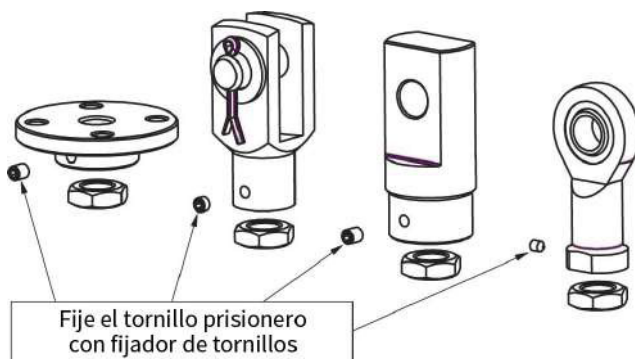
Fig. 9. Fije los accesorios como las bridas de sujeción, los cabezales de horquilla, rótula o pivotante después de ajustar la posición.
