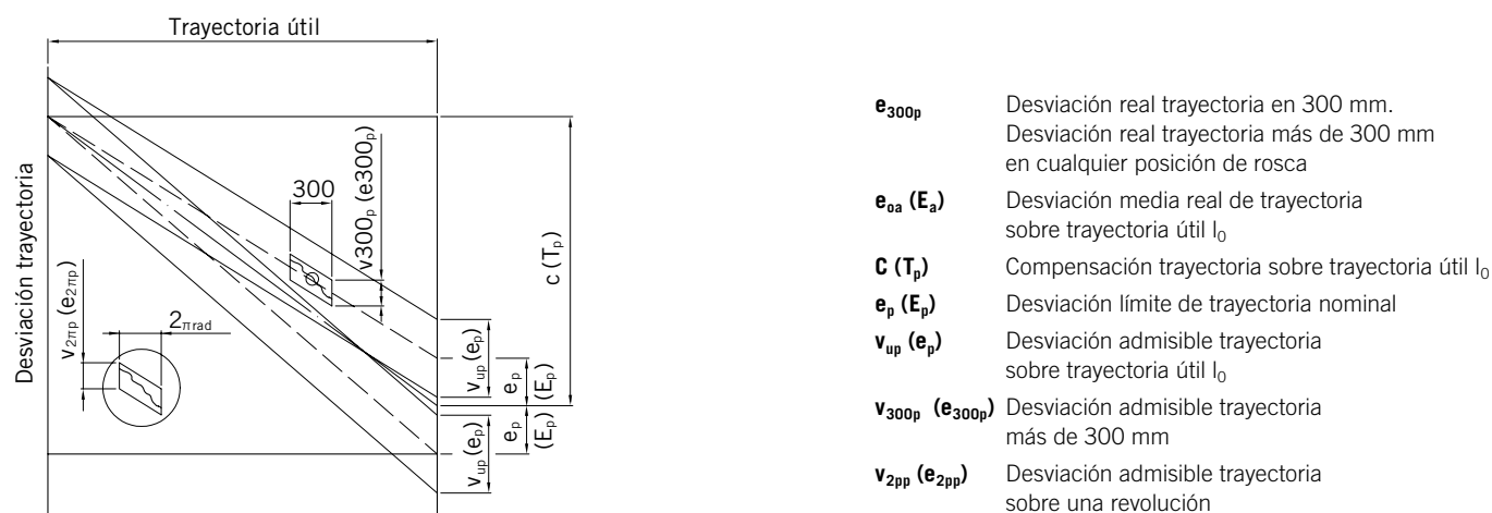
Fig. 3.11 Medición ISO DIN curva de paso del husillo de bolas
